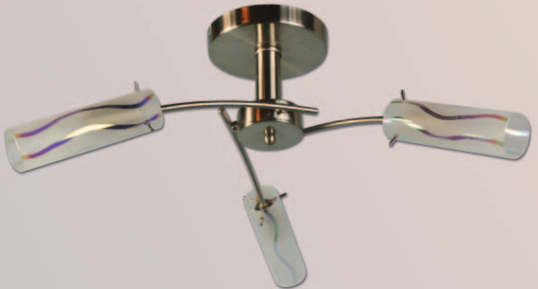
10104/3 ↓ 26, ↔ 42 3xE14 / 60W
