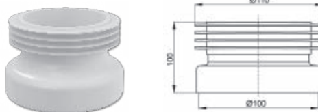
Эксцентрик резиновый (манжета) Alca Plast угловой A990
